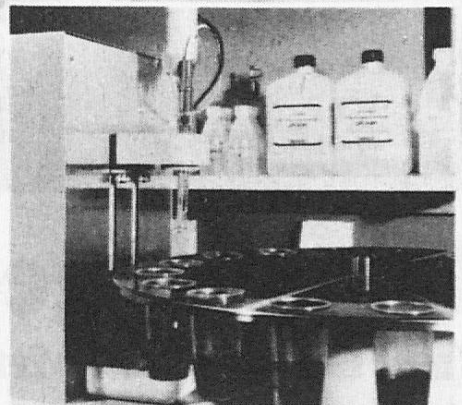
Probenwechsler RT40 mit 16 Probenplätzen für Kleinserien.
