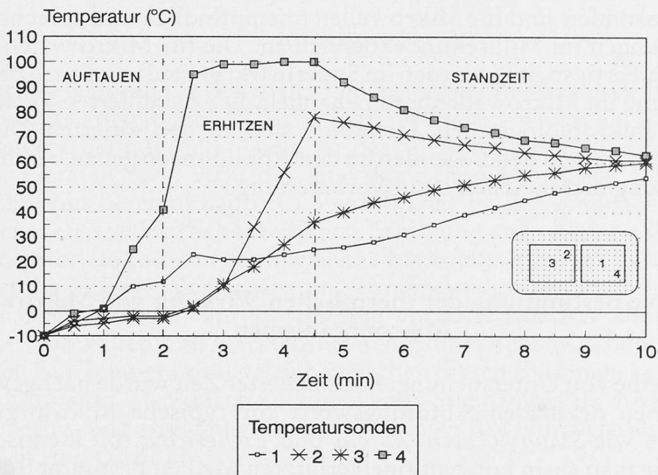
Abb. 1. Temperaturverlauf in 2 Rindfleischwürfeln von 4 cm Kantenlänge während Erhitzung in einem Mikrowellenofen. Die tiefgefrorenen Stücke ( -18^{\circ}\text{C} ) wurden im Zentrum des Herdes plaziert. Die Thermosonden (No. 1 bis 4) wurden wie angegeben von oben her 2 cm tief eingesetzt. In der Auftauphase gibt das Gerät 50% Leistung ab, während des Erhitzens 100%. In der Standzeit ist das Magnetron nicht im Betrieb. Das Fleischstück, das die Sonden 1 und 4 enthielt, wurde auf der Oberfläche mit Salz bestreut.
