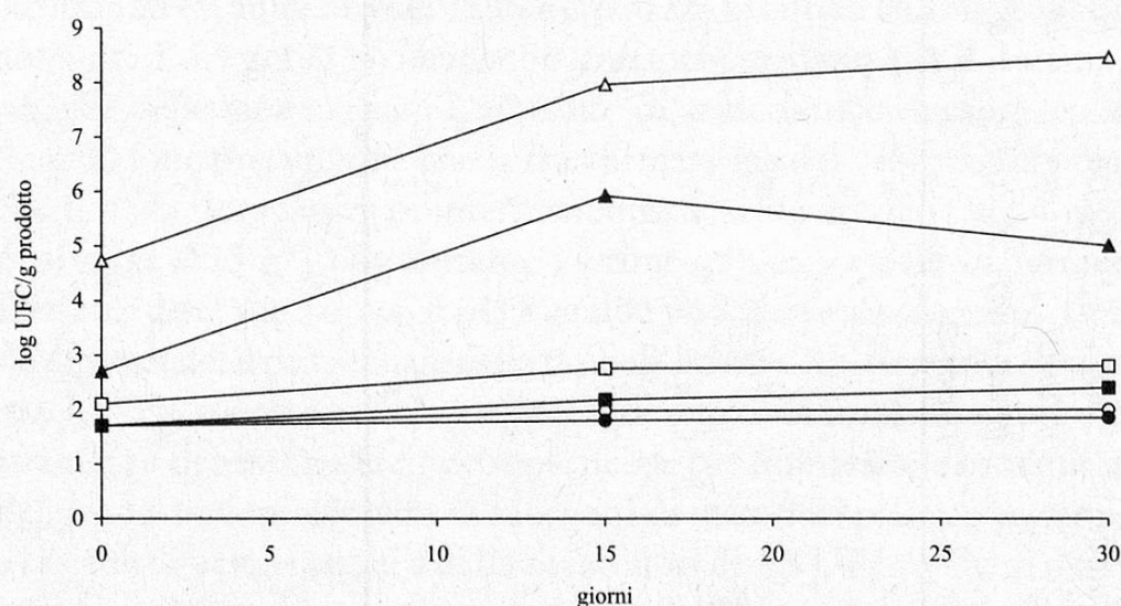
Figura 5 Evoluzione dei batteri lattici e dei lieviti a diversi trattamenti di pastorizzazione superficiale a 80 °C: sviluppo di batteri lattici (△) e di lieviti (▲) del sacchetto confezionato non pastorizzato; sviluppo di batteri lattici (□) e di lieviti (■) dopo pastorizzazione superficiale per 10 min del sacchetto confezionato; sviluppo di batteri lattici (○) e di lieviti (●) dopo pastorizzazione superficiale per 15 min del sacchetto confezionato.
