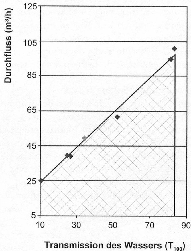
Abbildung 1 Dimensionierungskurve für eine UV-Desinfektionsanlage (T 100 : % Transmission bei 254,7 nm und 100 mm Schichtdicke) . Die Punkte stellen die im Rahmen der Zertifizierung gemessenen Betriebspunkte dar. Der grau unterlegte Bereich stellt somit Kombinationen aus Durchflusswerten und UV-Transmissionen dar, die eine minimale Dosis von 400 J/m 2 sicherstellen
