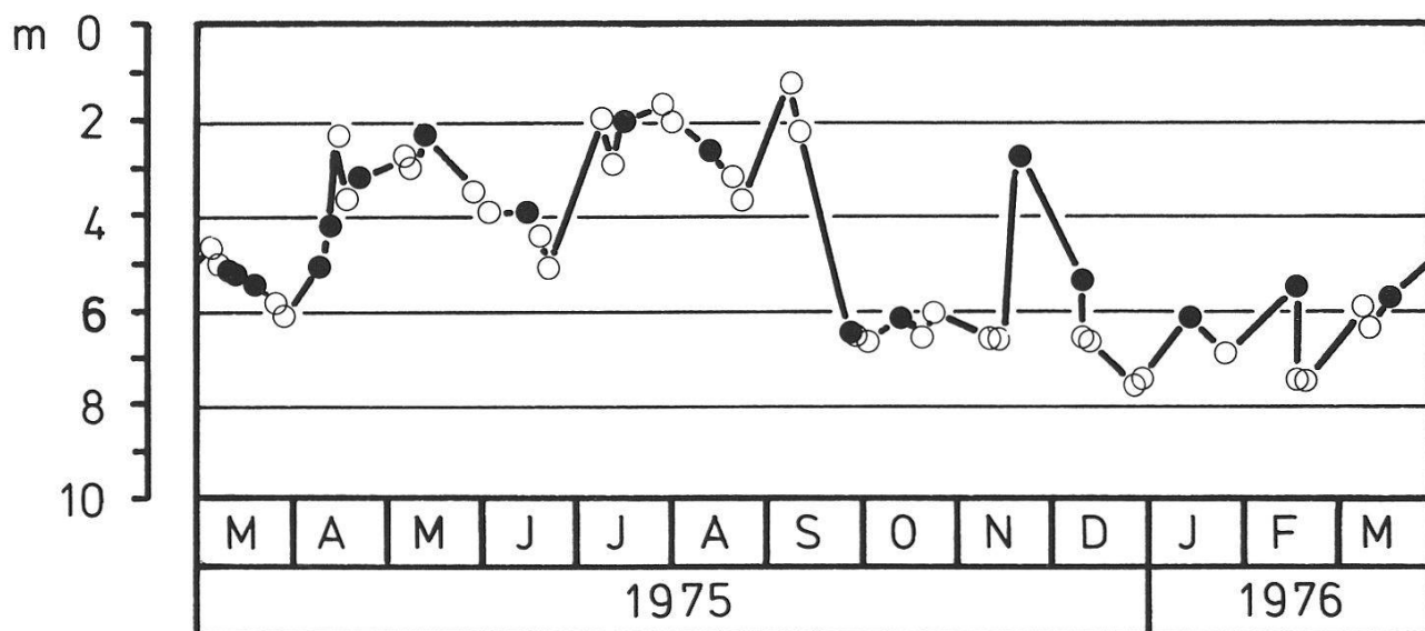
Abb. 3: Bielersee: Sichttiefen
