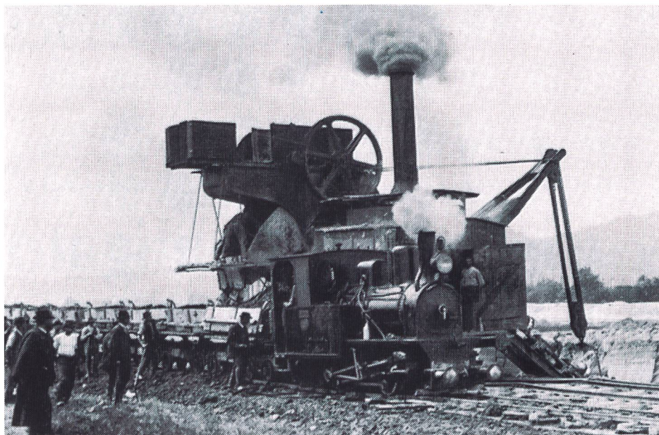
Lavori di scavo del canale per la regolazione del Reno, a Fussach, nel 1898, con una gigantesca scavatrice che carica il materiale sui vagoni.
