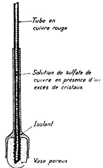
FIG. 12. — Electrode impolarisable type Schlumberger.
