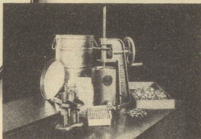
Apparatur zum Abfüllen der Tuben mit Spezialfett
