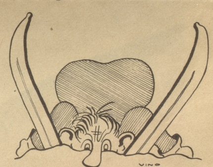
Der „Ski-Saurier“!
