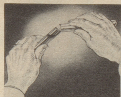
Jeder Chemiker kann das Vorhandensein des Tryptophan im Neo-Silvikrin mit Hilfe der Glyoxylsäure und H 2 SO 4 feststellen.
