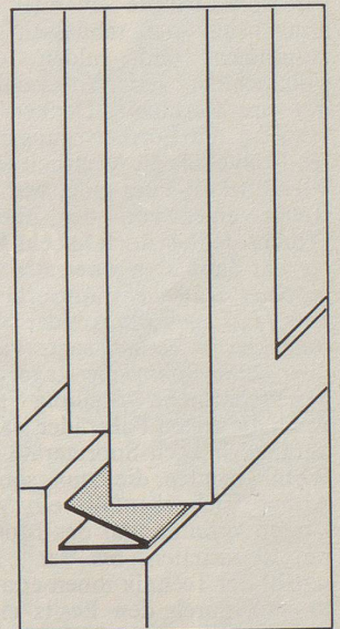
Scotch Weatherstrip: ein bewegliches «V», dessen Winkel sich als Windfänger der Breite von Fugen und Spalten massgerecht anpasst. Wo keine Zugluft durchkommt, weht auch kein Luftzug.
