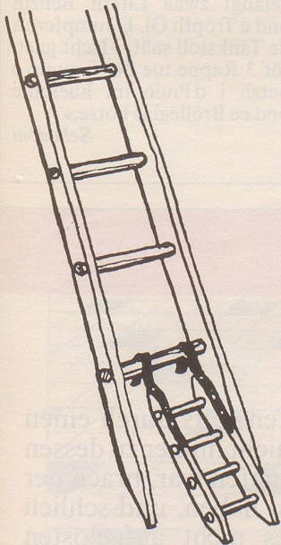
Haupt- und Hilfsleiter
