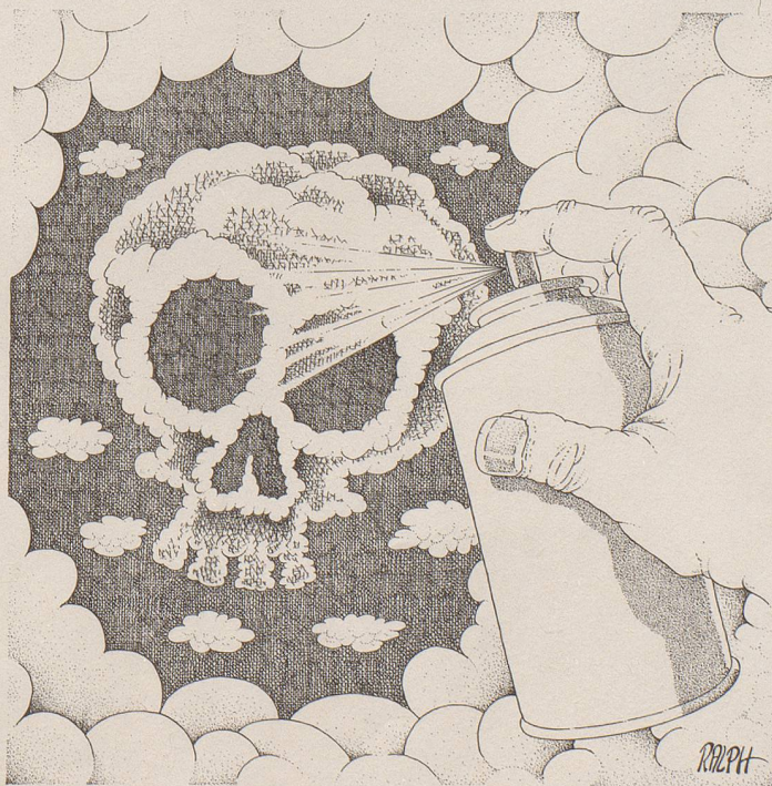
Das Ozonloch
