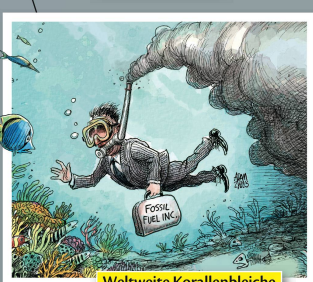
Weltweite Korallenbleiche
