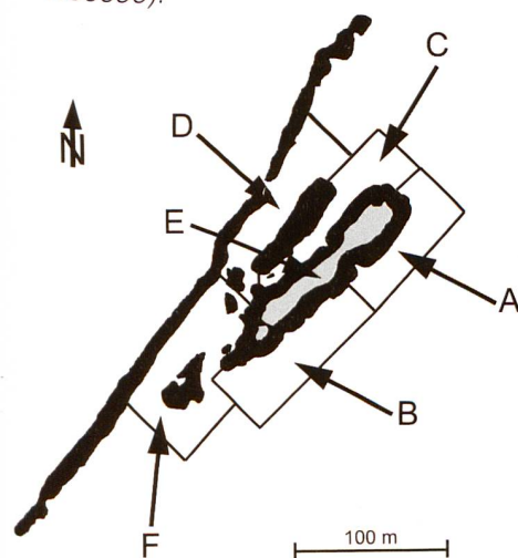
Abb. 3: Anordnung der sechs Sektoren A-F für die Untersuchung der Vielfalt der Moose, Gefässpflanzen und Landschnecken.
