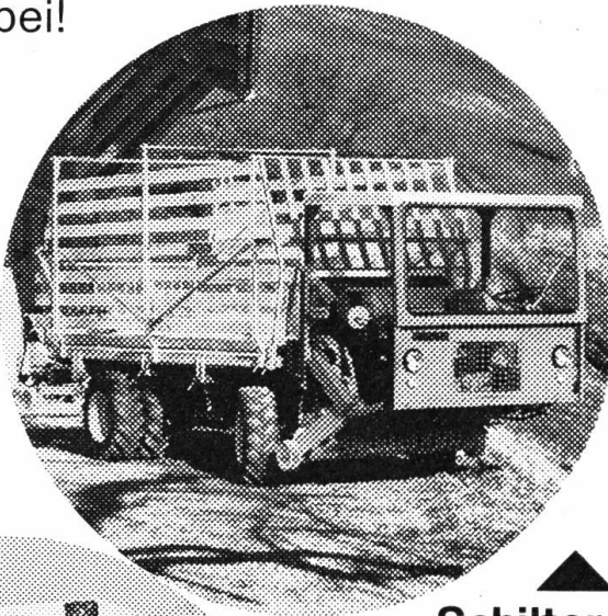
Schilter-Ladetraktoren: LT1 11 m 3 40 PS LT2 14 m 3 40 PS LT3 17 m 3 40 PS
