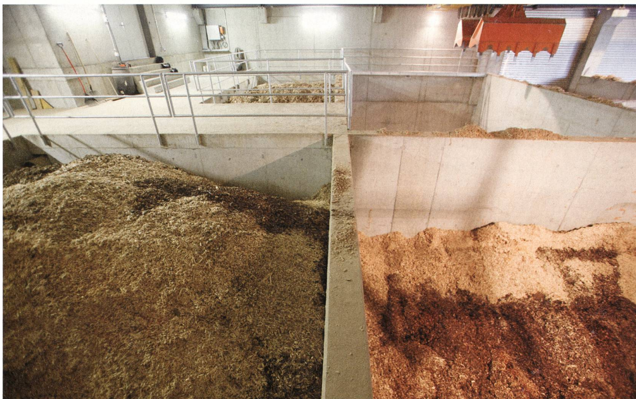
Blick ins Schnitzellager mit den Schubböden und dem ferngesteuerten automatischen Kran, der das Schnitzellager «bewirtschaftet».
