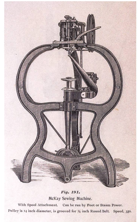
Abb. 6: Blake/McKay Maschine. Nähmaschinen ermöglichten ab ca. 1860 die Industrialisierung der Schuhmacherei. Vor allen die Einführung dieser amerikanischen Blake/McKay Maschine, die Sohlen direkt an den Schaft nähen konnte, bedeutete um 1870 einen Wendepunkt. © Sammlung Ballyana
