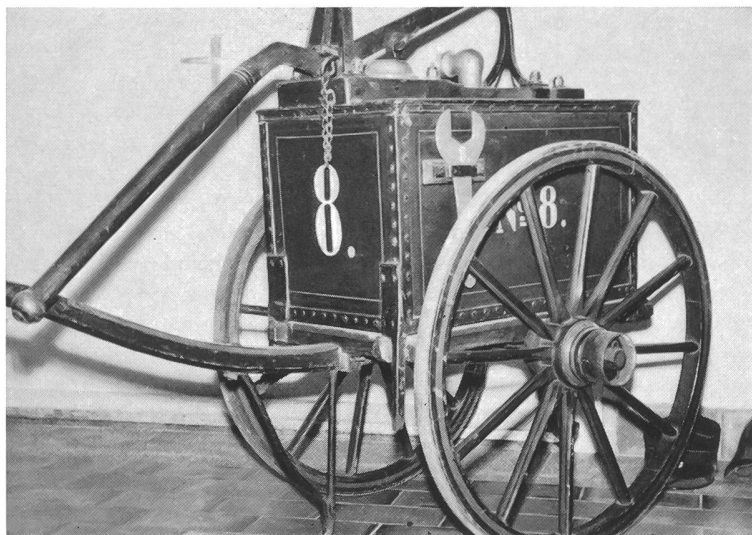
Fahrbare Handdruckspritze Olten aus dem 18. Jahrhundert (Hist. Museum Olten).
