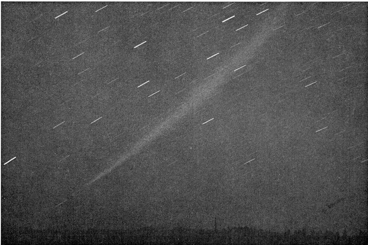
Fig. 3: Komet IKEYA-SEKI (1965 f). Aufnahme von MARTIN DUBS, Arbon, am 7. 11. 1965 5 km südlich von Heiden, 1089 m ü. M. mit Edixa-Kleinbildkamera-Optik 1:2.8, f = 50 mm, ohne Nachführung. Aufnahme von 5 h 45 min bis 5 h 50 min MEZ. Schweiflänge: visuell ca. 20°, photographisch ca. 28°. Schweifhelligkeit etwa gleich jener des Zodiakallichts. Atmosphärische Bedingungen: sehr gut.
