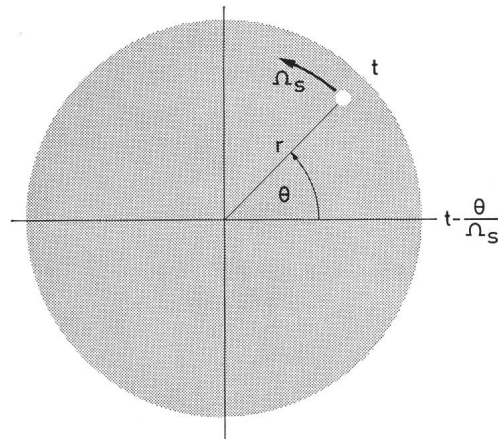
Fig. 3: Im Abstand r mit der Winkelgeschwindigkeit \Omega_s umlaufende Störung.
