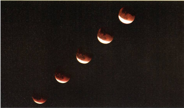
Abb. 1 Totale Mondfinsternis vom 28. Oktober 1985, kurz nach Ende der Totalität um 19.05 h MEZ. Aufnahmezeiten: 19.11.00 / 19.14.30 / 19.18.00 / 19.21.30 / 19.25.00 MEZ. - Dia-Film Fujichrome DX 400, Teleobjektiv 400 mm, Blende 11, Belichtungszeiten je ca. 1,5 Sekunden.
