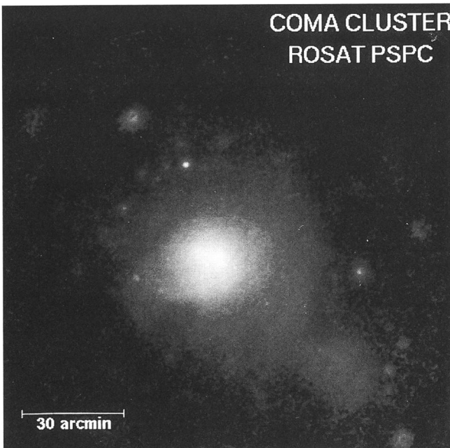
5. Vereinigung des Komahaufens mit einem kleineren Galaxienhaufen, der von rechts unten einfällt.
