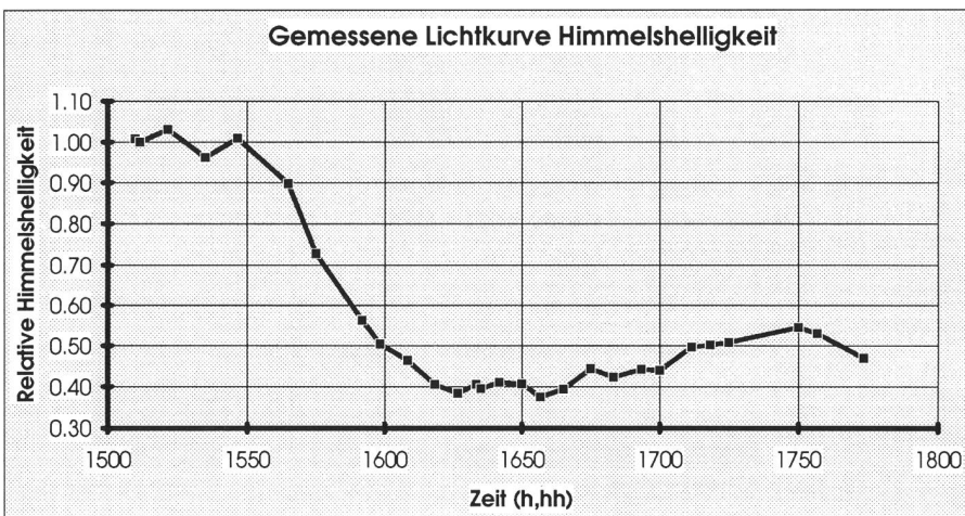
Diagramm 2: Gemessene Lichtkurve der Himmeshelligkeit
