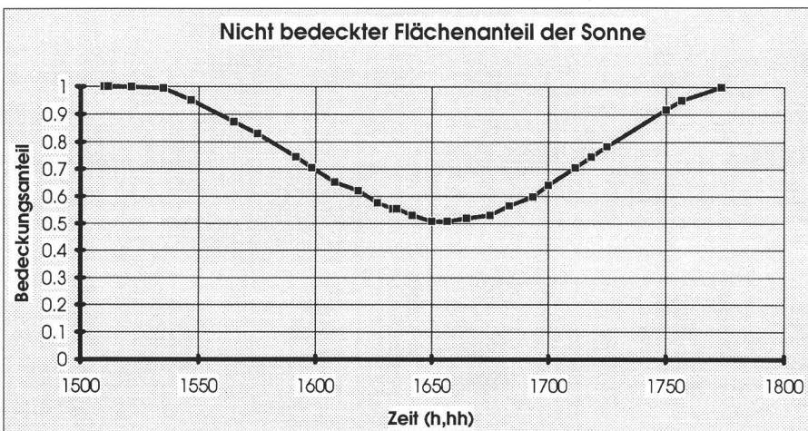
Diagramm 3: Theoretische Lichtkurve der Himmeshelligkeit (Bedeckungsanteil der Sonne)
