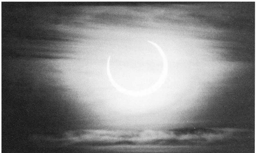
Fig. 3: Bereits anderthalb Minuten nach Ende der Ringphase leuchtete nur 3^\circ hoch über dem Horizont eine schlanke Lichtsichel über der Taddla-Ebene.
