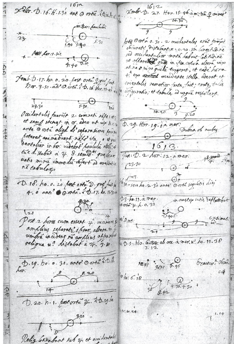
Fig. 2: Observations des satellites de Jupiter faites par Galilée en décembre 1612 et janvier 1613. Les lunes sont identifiées par le nombre de points: Callisto (3), Ganymède (2), Europe (1) et Io (0) (de The Cambridge Atlas of Astronomy , third edition).
