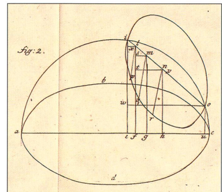
Fig. 10: Zweite Figur zu DANIEL BERNOULLIS Abhandlung über die Polhöhenbestimmung. Die Kreise abcd und ipqro stellen den Horizont sowie einen Deklinationskreis dar, der Halbkreis aioc ist der Ortsmeridian. p, q und r sind die gemessenen Sternhöhen.
