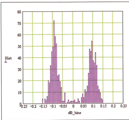
Fig. 4: Histogram der Daten aus dem File aus Fig. 3 oben. Die Funktion links im Bild zeigt die Verteilung der Hintergrundstrahlung, während die Funktion rechts die Verteilung der Mondradiostrahlung inklusive Hintergrund zeigt. Der Unterschied beider Funktionen wird gespeichert als Einzelwert ausgedrückt in Dezibel, hier im vorliegenden Beispiel sind es etwa 0.197dB, entsprechend einer Antennentemperatur von etwa 4.4 Kelvin, dies bei einer mittleren Systemtemperatur von etwa 94 Kelvin.
