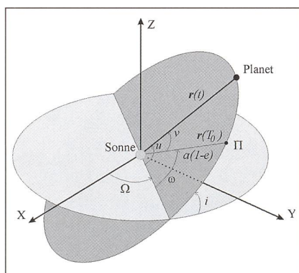
Fig. 1: Keplersche Bahnelemente.
