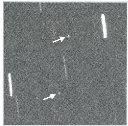
Fig. 7: Kleiner Ausschnitt aus einer Suchaufnahme von Teneriffa. Die mit Pfeilen markierten Objekte (astronomische Helligkeit m_v = 19 ) sind kleine Schrotteile von ca. 30 Zentimetern Durchmesser in einem Abstand von 36 000 Kilometern!
