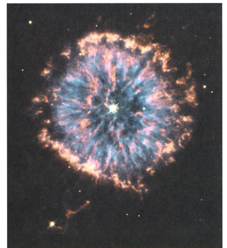
Fig. 4. La nébuleuse planétaire NGC6751 (© STScI)
