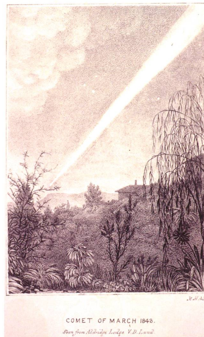
Abbildung 6: Der «Grosse Komet 1843», gesehen in Australien. Er tauchte im März 1843 auf und kam der Sonne mit einer Periheldistanz von bloss 830'000 km extrem nahe! Er war so hell, dass man ihn 1^\circ neben der Sonne bei Tag sehen konnte. Dieser Komet zeigte, dass auch C/2012 S1 (ISON) mit einer doch beachtlichen Annäherung an das Tagesgestirn von 1,8 Millionen km durchaus «überleben» könnte! Sollte dies der Fall sein, wäre uns eine spektakuläre Kometenerscheinung sicher. (Quelle: Wikipedia)
