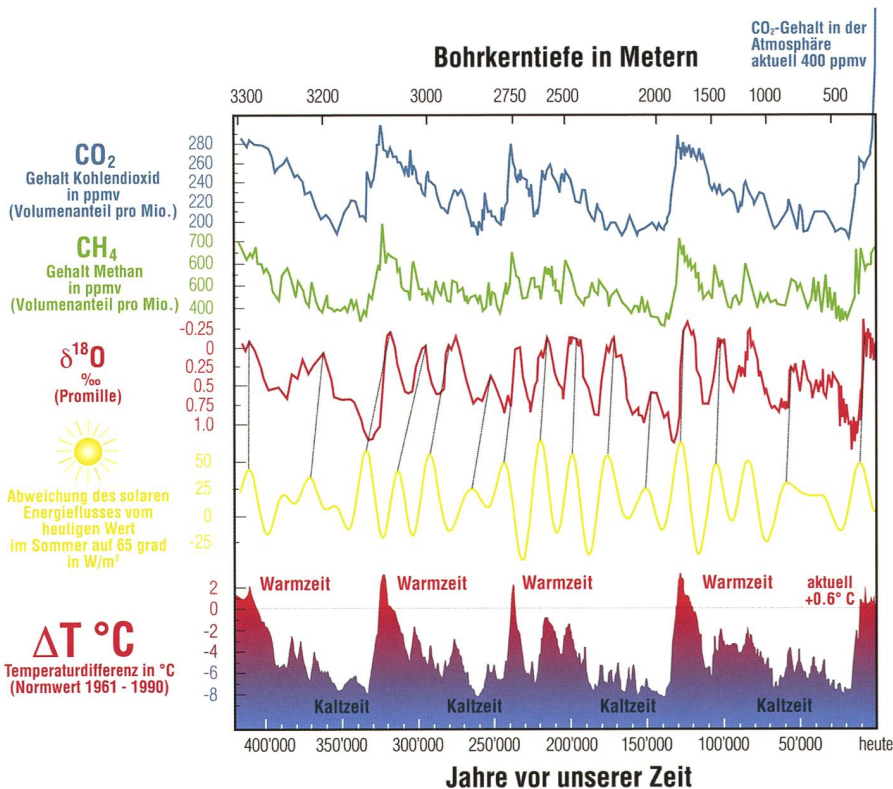
Abbildung 8: Aus Eisbohrkernen bis zu 3,5 Kilometer Tiefe kann die Erdklimageschichte bis 400'000 Jahre vor heute zurückverfolgt werden. Wir sehen die natürlichen Schwankungen des CO 2 , CH 4 und 18 O-Gehaltes, sowie den sich ändernden solaren Energiefluss, bedingt durch die MILANKOVIĆ-Zyklen auf dem 65. nördlichen Breitenkreis. Auffällig ist die Korrelation mit den Temperaturabweichungen (ganz unten). Trotz des anthropogenen CO 2 -Ausstosses um fast 120 ppm über den «natürlichen Spitzen» liegt die globale Temperaturabweichung aktuell bei +0.6°C. Wie wir sehen, lagen die Temperaturen früherer Warmzeiten über dem heutigen Wert! (Grafik: Thomas Baer)
