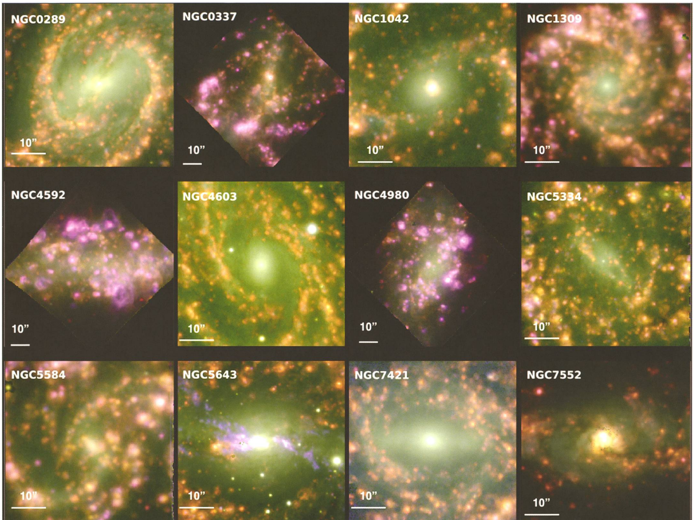
Abbildung 5: Diese Aufnahmen vom MUSE-Instrument zeigen Spiralgalaxien in unserer Umgebung. In den Farben wird das ionisierte Gas gezeigt, insbesondere in rot die H\alpha -Emissionslinie, in grün die [SII] -Emissionslinie und in blau die [OIII] -Emissionslinie. Die Belichtungszeit beträgt ca. 1 Stunde. Diese Aufnahmen entstanden im Sommer 2015 als Teil von «MUSE Atlas of Disks», ein Projekt, das von der ETH geleitet wird, und die physikalischen Prozesse rund um die Sternentstehung in Galaxien beantworten soll.
