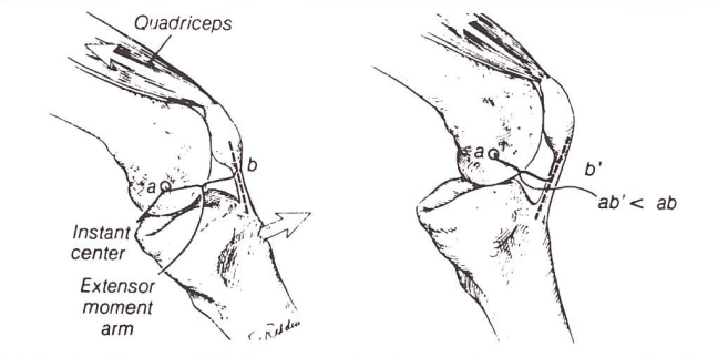
Fig. 5: Der Momentarm der Lig. patellae, bis die aktuelle Rotationsachse (instant center) bestimmt wird durch die Translationsrichtung der Tibia beim Quadricepsstraining. (1980, Baylor College of Medicine. Cain T.E. Performance of an athlete with straight posterior knee instability the am jour. of sp. med. vol. 9 no. 4 fig. 8)
