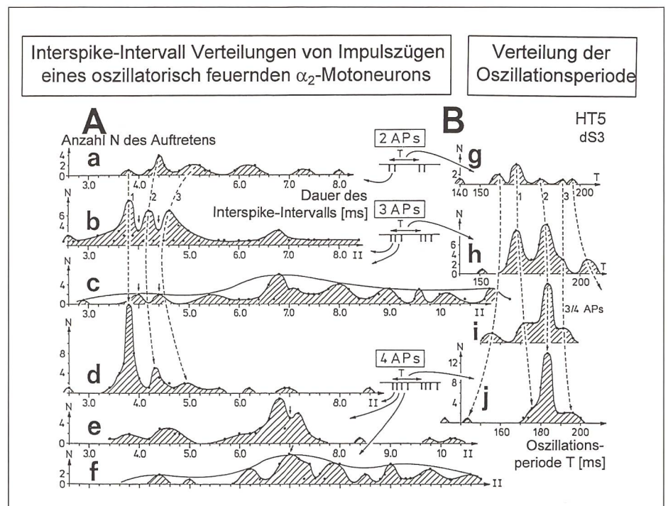
Abb. 20: Interspike-Intervall-Verteilungen der Impulszüge (A) und der korrespondierenden Oszillationsperioden-Verteilungen (B) für verschiedene Impulszug-Längen.
