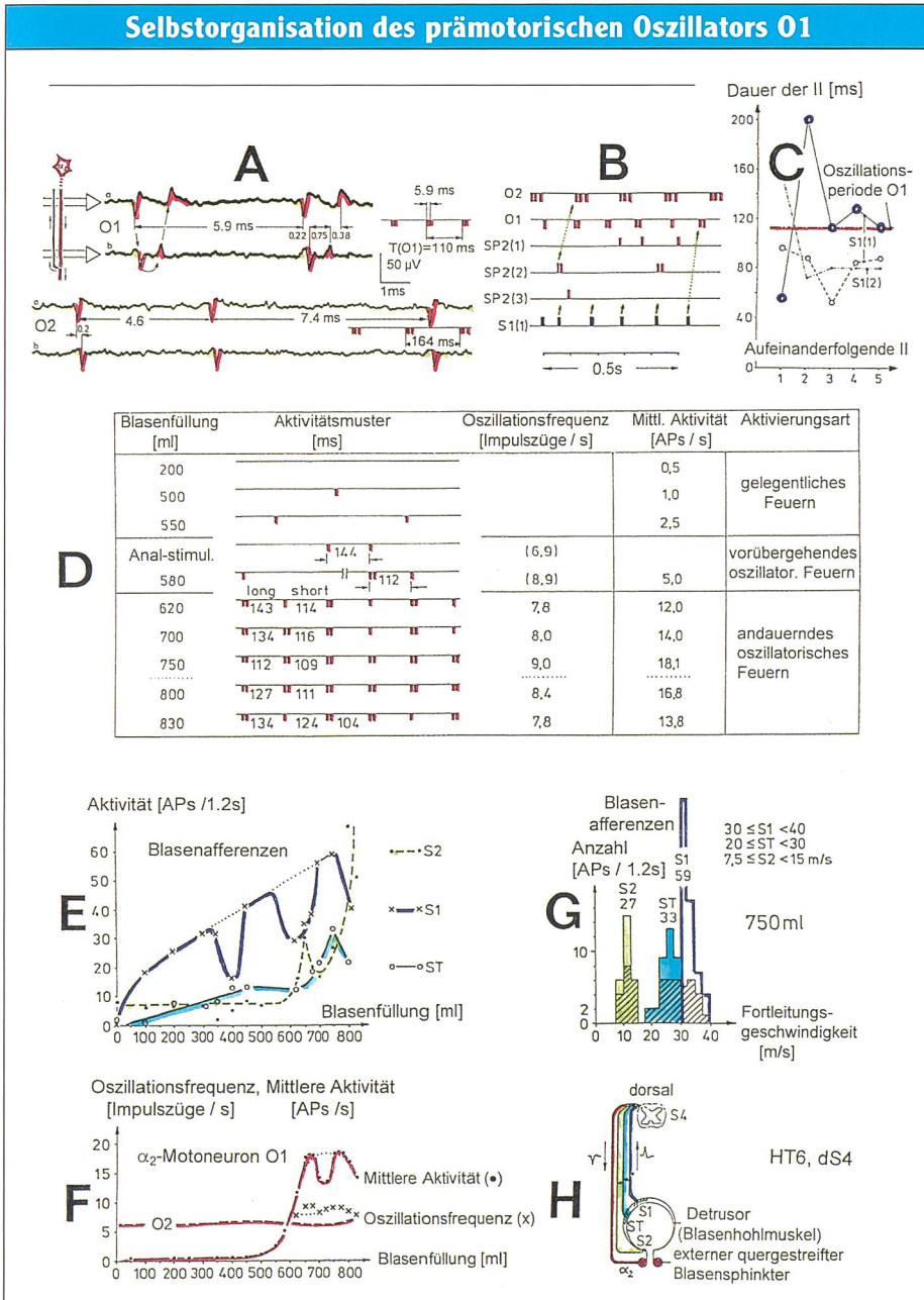
Abb. 19: Selbstorganisation des prämotorischen \alpha_2 -Oszillators O1, welcher den quergestreiften externen Blasenphinkter innerviert und aktiviert. Hirntoter HT6. Ableitung von einer dorsalen S4 Nervenwurzel.
