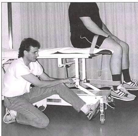
Abbildung 4: Isometrische Kraftmessung der Knieextension mit der Kraftmesszelle nach Huber et al. (Huber et al. 1997).
