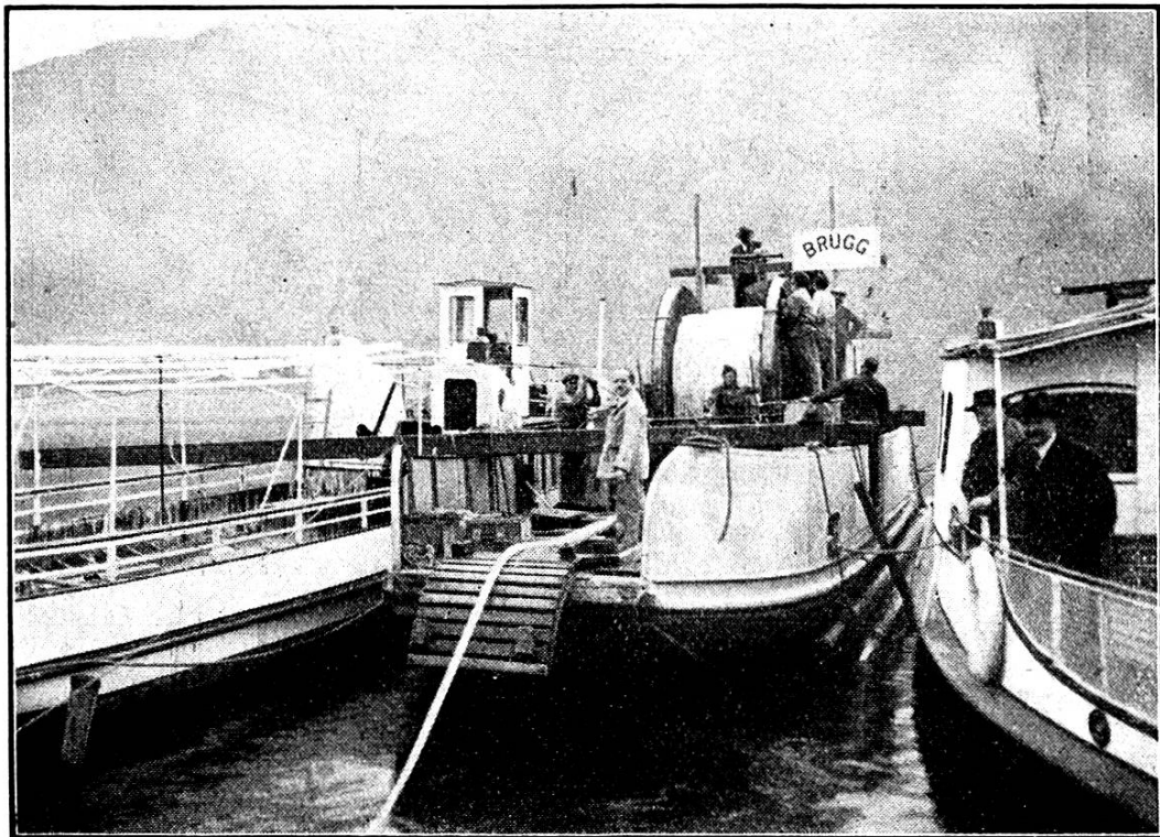
Verlegung im November 1934 eines Telephonkabels im Luganersee zwischen Mor-cote und Brusino für die Post- und Telegraphenverwaltung.
