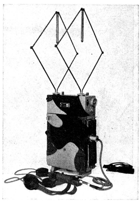
Tragbares Gerät für drahtlose Telephonie mit Dezimeterwellen
