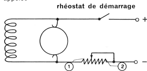
fig. 138 1 Marche 2 Démarrage
