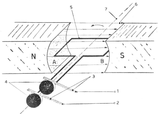
Fig. 142 1 und 2 Anschlussklemmen 5 Drahring (Schleife) 3 Bürsten 6 Pollinie 4 Schleifringe 7 Achse
