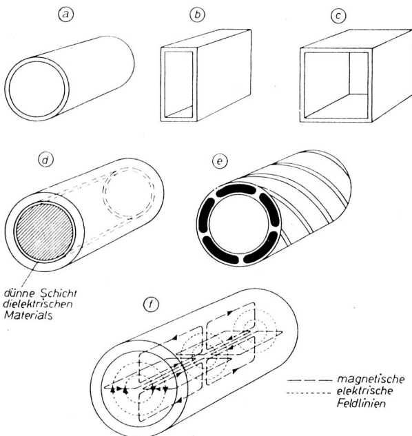
Hohlleiter mit rundem (a), rechteckigem (b) und quadratischem (c) Querschnitt; zur Unterdrückung unerwünschter Wellentypen mit dielektrischem Material bedeckt (d) oder aus Wenden aufgebaut (e); Feldlinien der H_{01} -Welle im Hohlleiter mit rundem Querschnitt (f).
