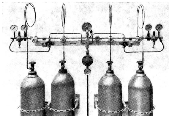
Stationäre Sauerstoff-Versorgungs-Zentrale
