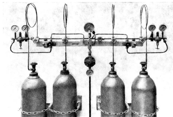
Stationäre Sauerstoff-Versorgungs-Zentrale
