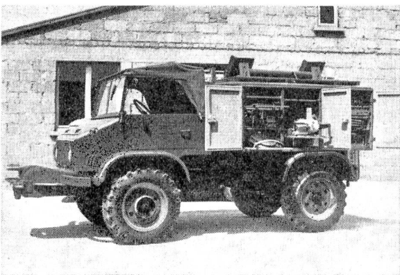
Rettungsdienstwagen mit UNIMOG-S-Fahrgestell
