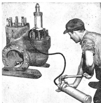
Hochdruck-Hydraulik (700 atü), kompakt gebaut, 9—900 t, mit oder ohne Zentrumloch
