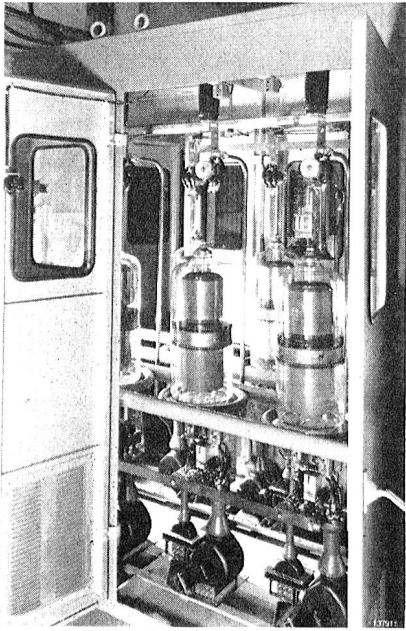
Teil eines Gleichrichterschrankes, mit sechs Hochleistungsthyratrons, die eine maximale Leistung von 19 kV/345 A abzugeben in der Lage sind. Der Gleichrichter dient zur Speisung von 500 kW bis 1000 kW Gross-Sendern.
