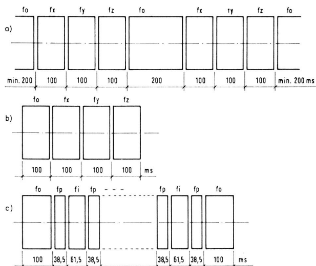
Fig. 2 a) Rufzeichen ( f_x, f_y, f_z : 3 Codefrequenzen/ f_0 : Freitonfrequenz während den Pausen) b) Teilnehmerkennzeichen ( f_y, f_x, f_z : 3 Codefrequenzen/ f_0 : Freitonfrequenz für Steuerimpuls) c) Wahlzeichen ( f_i : Frequenz für Wahlimpuls/ f_p : Frequenz für Wahlpause/ f_0 : Freitonfrequenz als Steuerimpuls)
