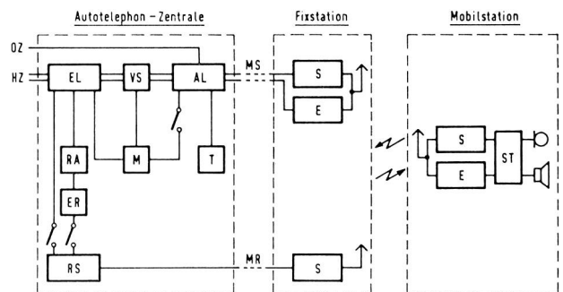
Fig. 3 Blockscha des funktionellen Zusammenwirkens der einzelnen Anlagenteile
