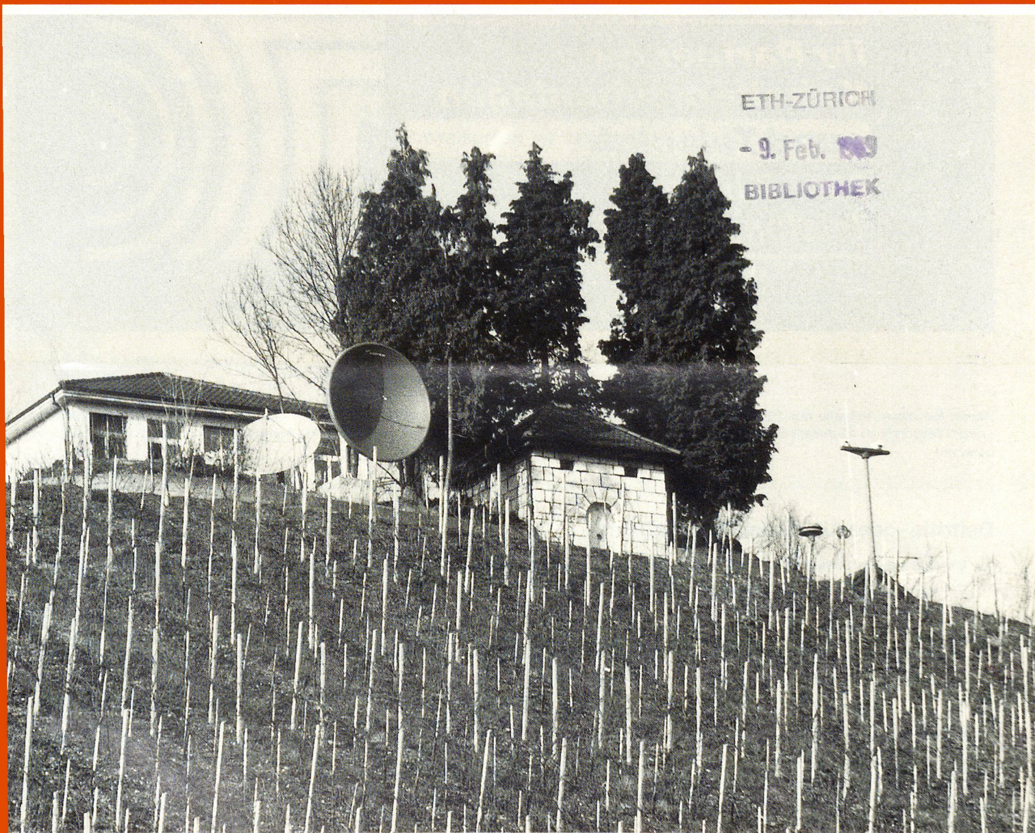
Grossgemeinschaftsantennenanlage Rheinau (Foto: R. Kilchmann)
