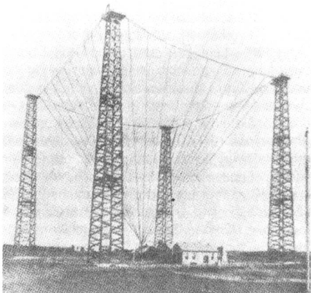
Fig. 2 Quadratische Pyramidenantenne in Marconis Poldhu-Station in England 1905. [15]
