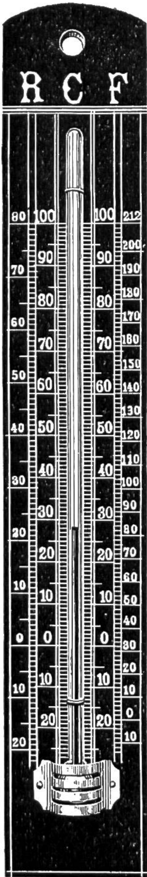
Réaumur-Celsius-Fahrenheit
